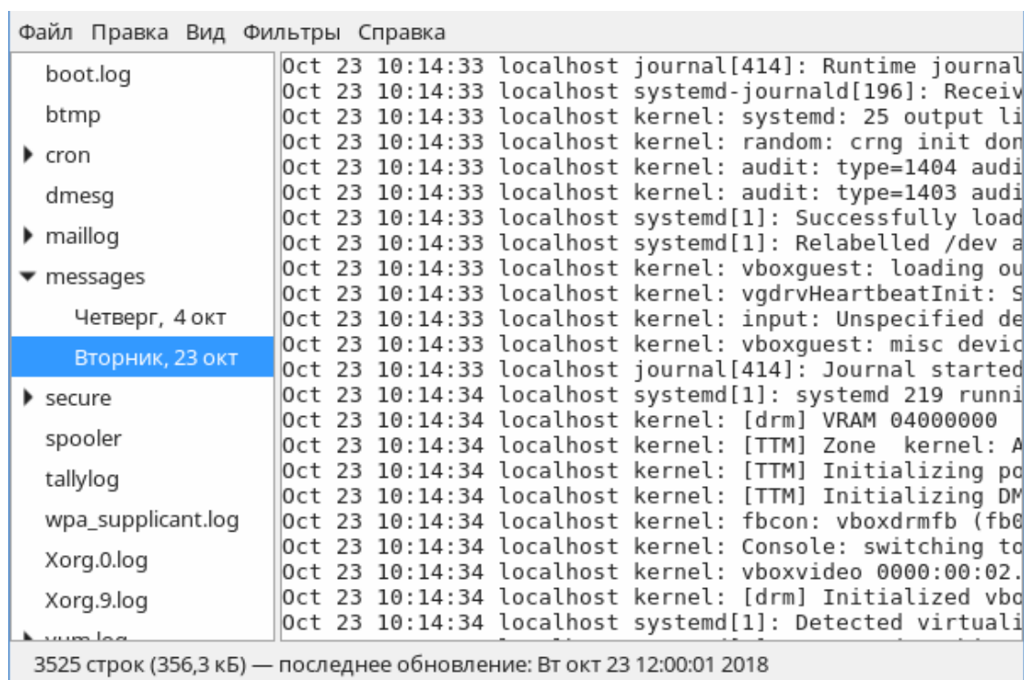
Рисунок 6.1 - Окно Программы просмотра системных журналов
