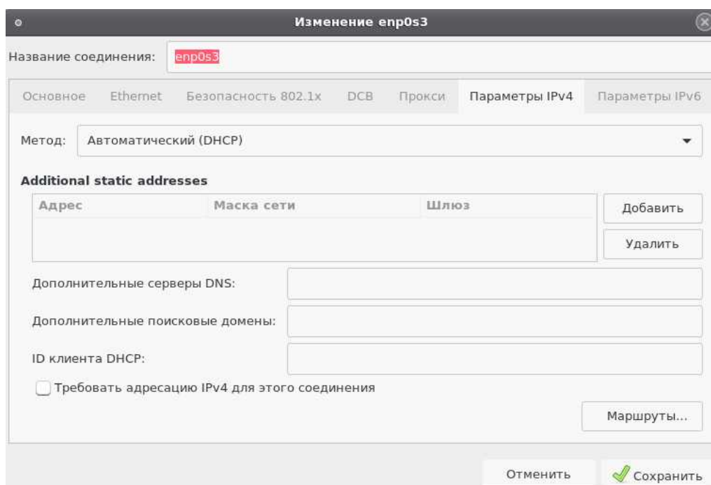
Рисунок 8.3 – Изменение свойств сетевого адаптера
